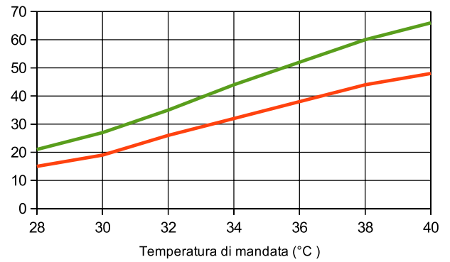
Rivestimento in legno 15 mm ( R=0,7 \text{ m}^2 \text{ k/W} )
